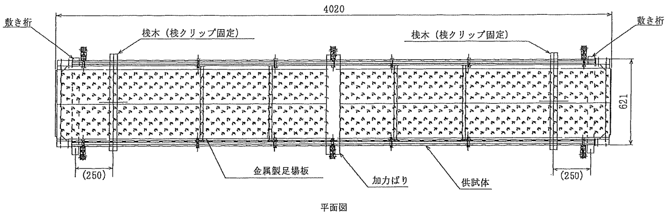
試験方法図1(①) : スタートインフレーム 型式 : FS-SF40Y
